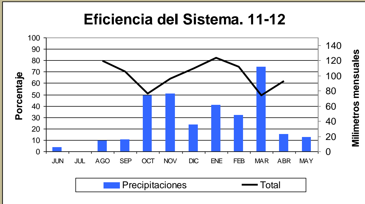
Gráfico 2, Eficiencia del sistema de riego
